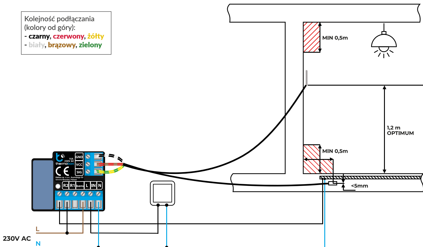
Schemat podłączenia mat grzewczych 230V:
